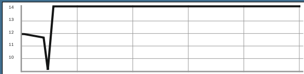
Diagramme de charge de la batterie pour les véhicules classiques
